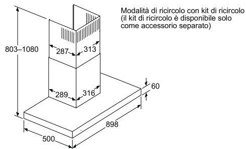
Prospettiva ricircolo
