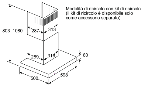
Prospettiva ricircolo
