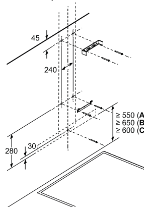
Installazione a parete con camino
