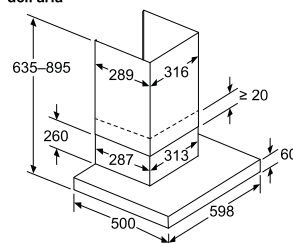
Apparecchio in modalità di estrazione dell'aria
